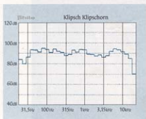
Abb. 1: Frequenzgang am Hörplatz
